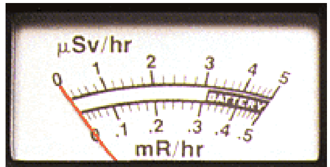
Optional SI Meter Scale: 0-500 µS/hr & 0-50 mR/hr
